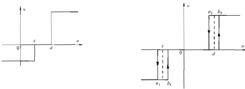
a) 无切换差的三位元件
