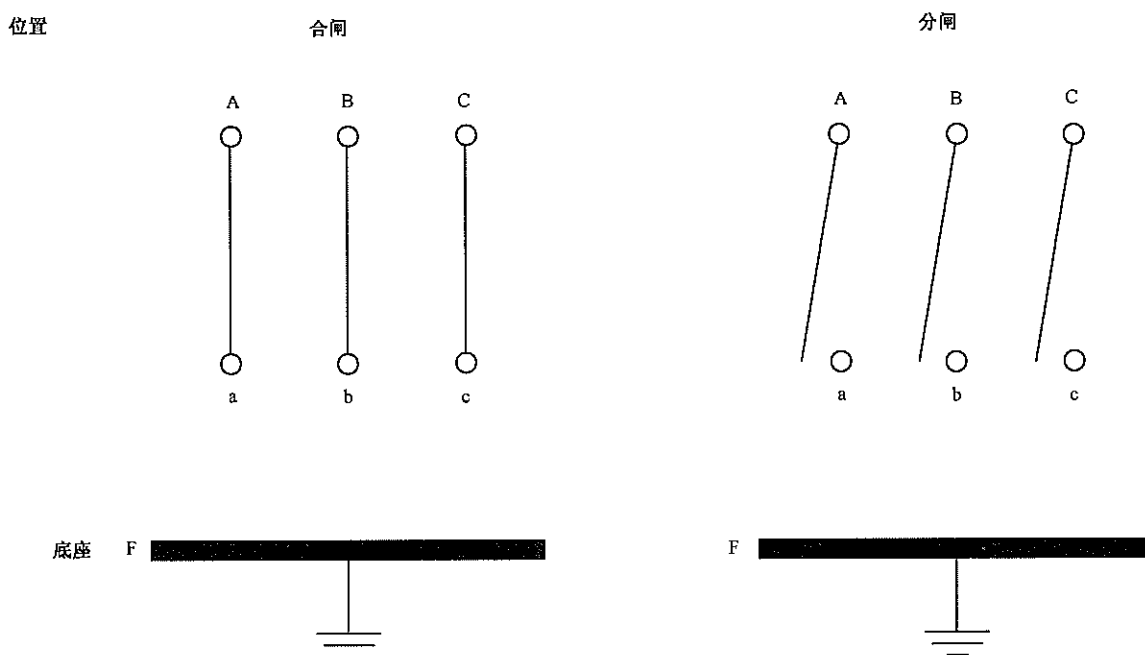
图 3 三极开关装置的联结图
