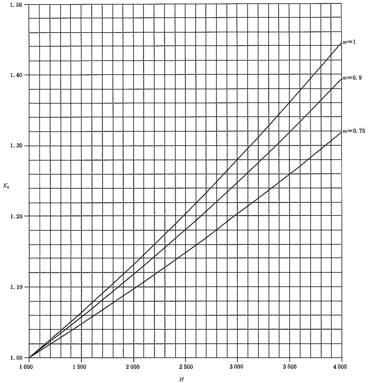
图 1 海拔修正系数
