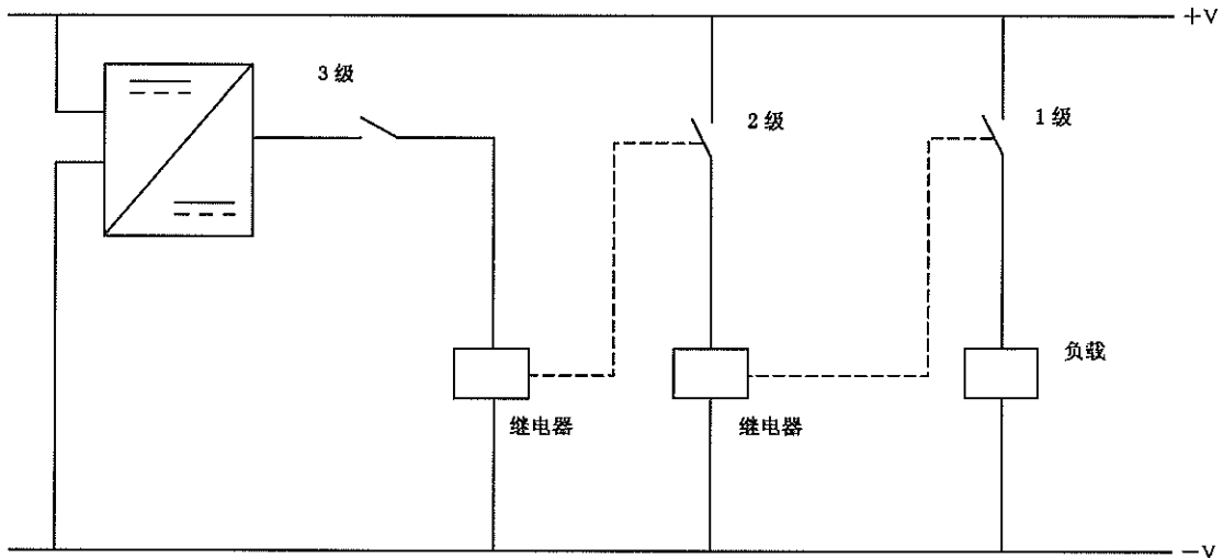
图 2 触头等级的例子
