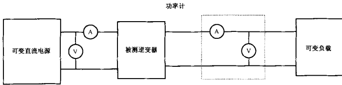
图 8 测试电路
